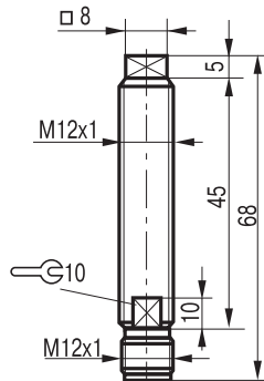
Габаритный чертёж
